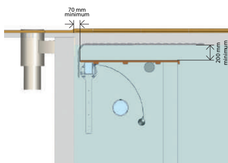
Dimensions d'installation système sous plage immergée
